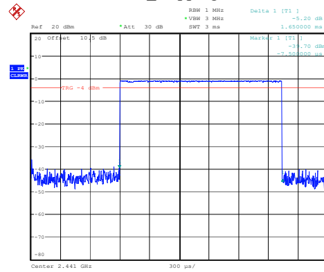
DH3_Hopping 1.650ms
