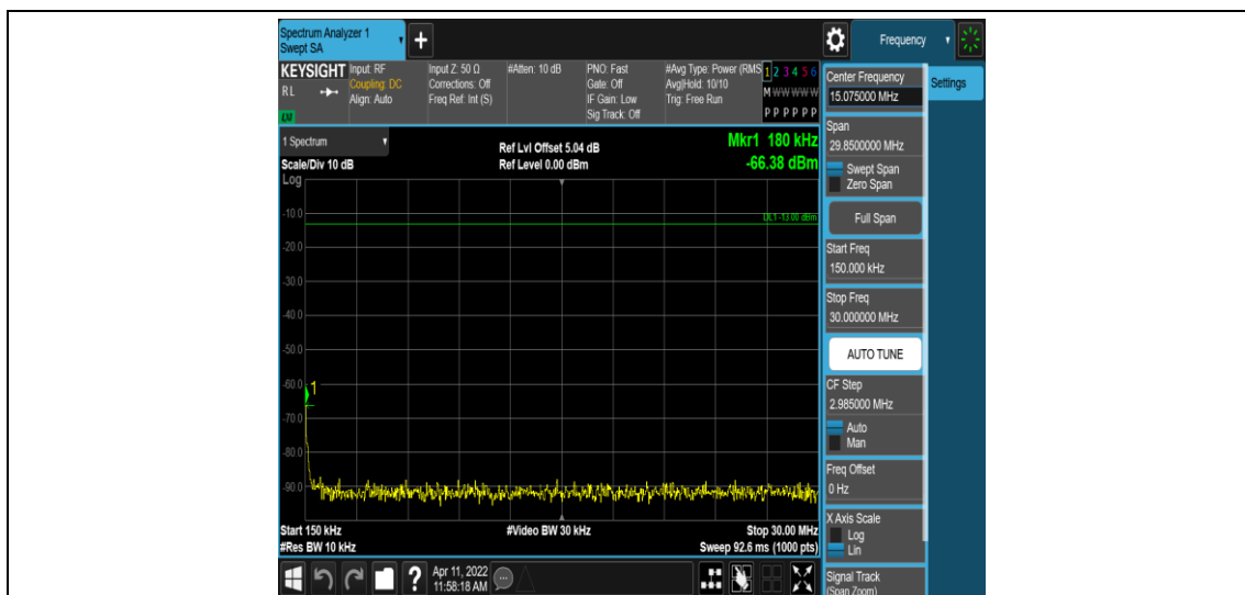
Band12-1.4MHz-QPSK-23173-1RB#0-Range2:0.15~30MHz
