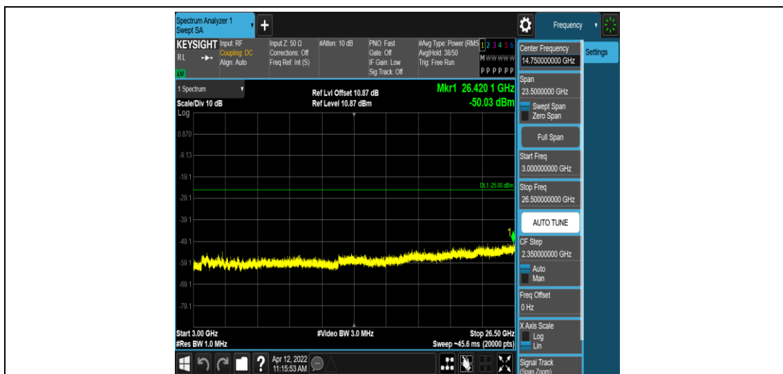
Band7-20MHz-QPSK-21350-1RB#0-Range5:3000~26500MHz
