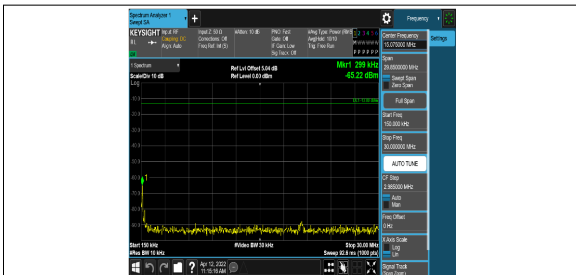
Band7-20MHz-QPSK-21350-1RB#0-Range2:0.15~30MHz
