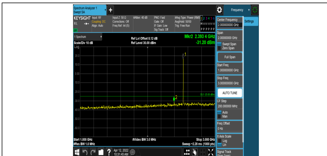
Band7-10MHz-QPSK-21100-1RB#0-Range4:1000~3000MHz
