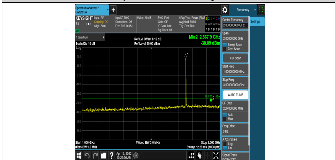
Band7-10MHz-QPSK-20800-1RB#0-Range4:1000~3000MHz
