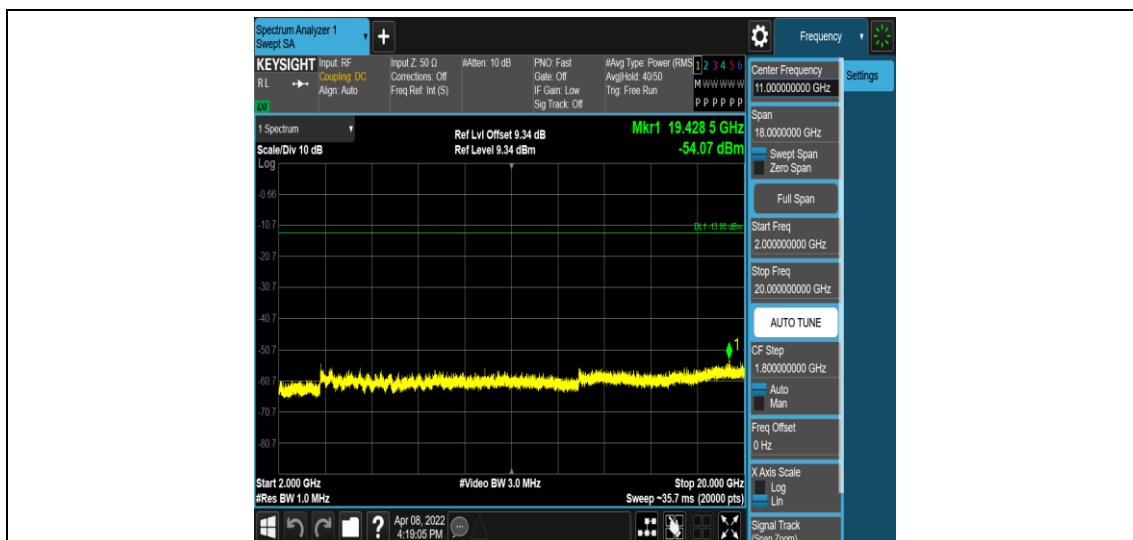
Band2-20MHz-QPSK-18700-1RB#0-Range5:2000~20000MHz
