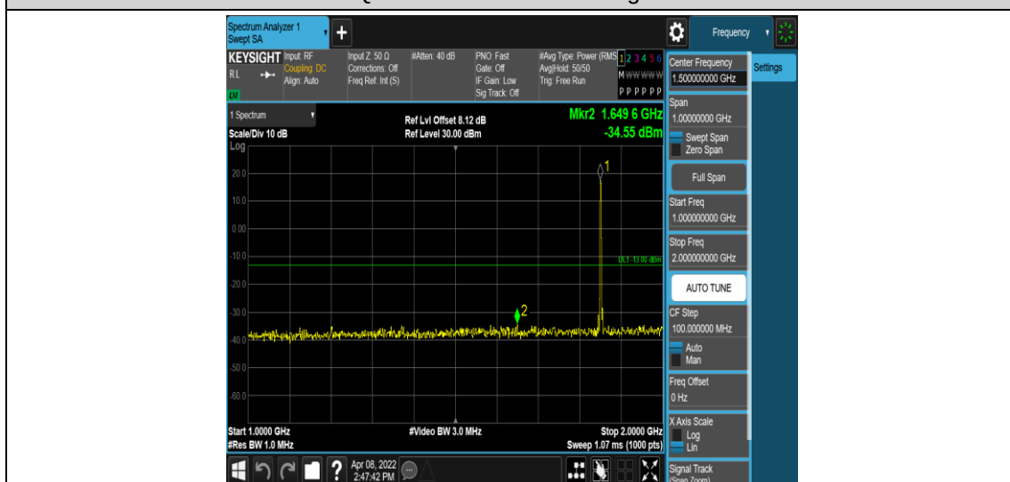
Band2-3MHz-QPSK-18615-1RB#0-Range4:1000~2000MHz
