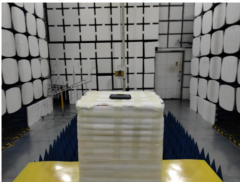
Fig. 2 (Above 1GHz)
