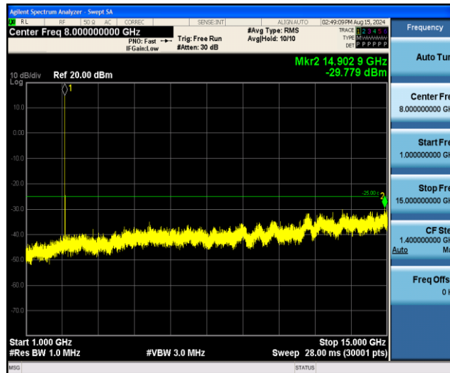
Band7-10MHz-QPSK-20800-1RB#0-Range2:1000~15000MHz
