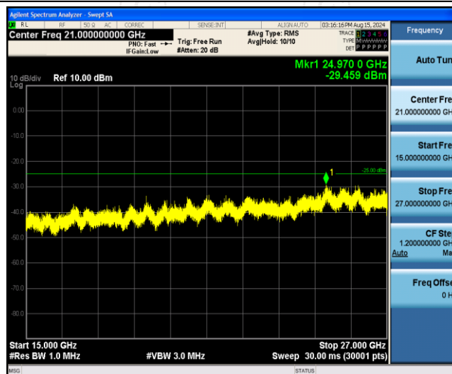
Band7-20MHz-QPSK-21100-1RB#0-Range3:15000~27000MHz
