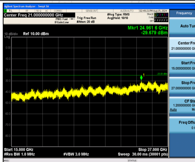
Band7-10MHz-QPSK-20800-1RB#0-Range3:15000~27000MHz
