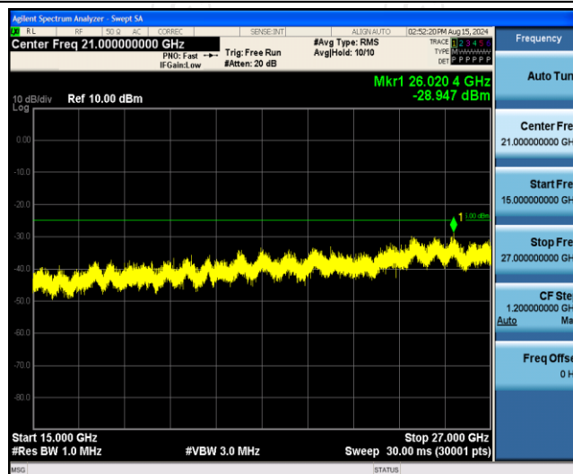
Band7-10MHz-QPSK-21400-1RB#0-Range3:15000~27000MHz
