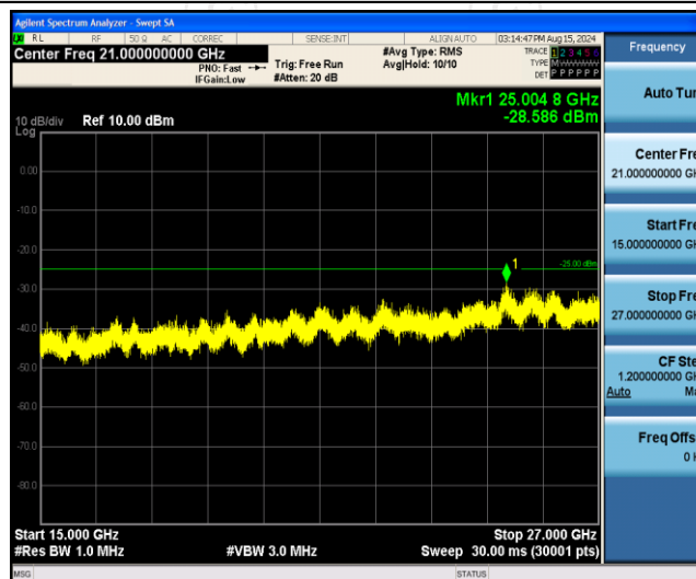
Band7-20MHz-QPSK-20850-1RB#0-Range3:15000~27000MHz
