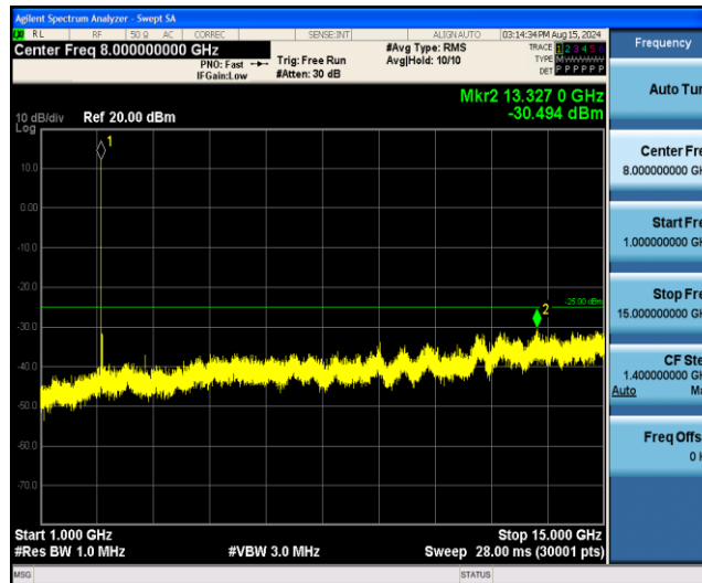
Band7-20MHz-QPSK-20850-1RB#0-Range2:1000~15000MHz
