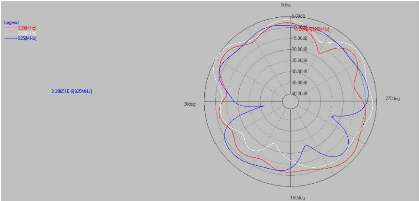
2D方向图
