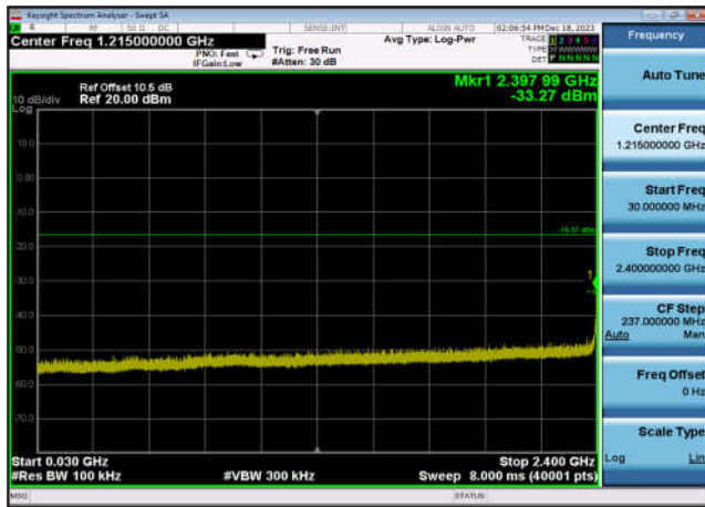
,Plot 3,30MHz~2400MHz-802.11ax(HE20) ,2462MHz,Ant0
