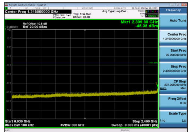
,Plot 3,30MHz~2400MHz-802.11ax(HE40) ,2452MHz,Ant0
