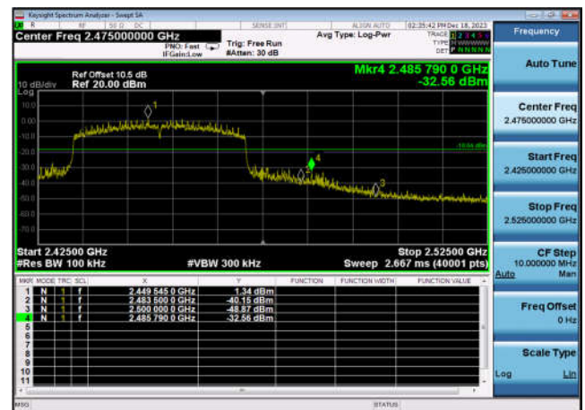
,Plot 2,Band Edge-802.11ax(HE40) ,2452MHz,Ant0
