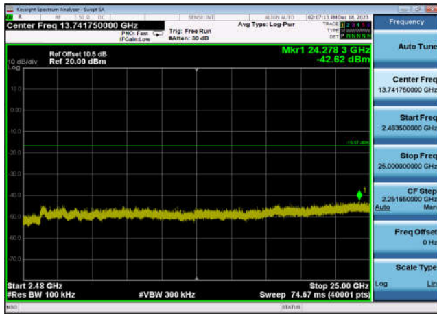
,Plot 4,2483.5MHz~25000MHz-802.11ax(H E20),2462MHz,Ant0
