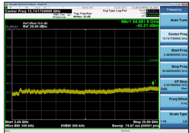
,Plot 4,2483.5MHz~25000MHz-802.11n(HT20),2462MHz,Ant0
