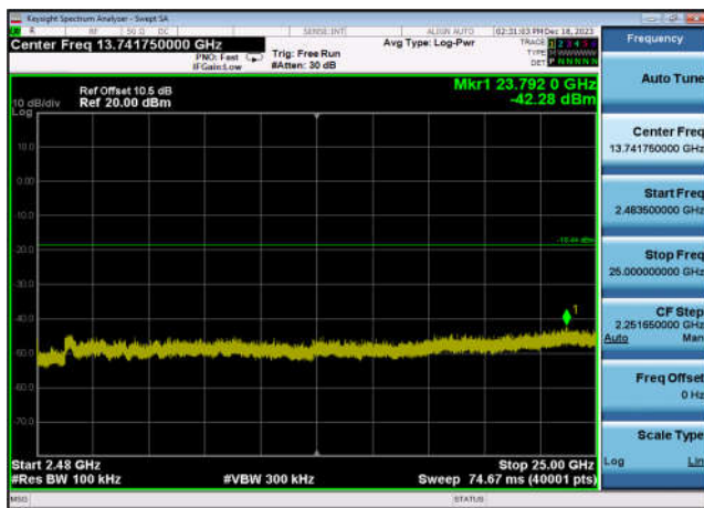
,Plot 4,2483.5MHz~25000MHz-802.11ax(H E40),2437MHz,Ant0
