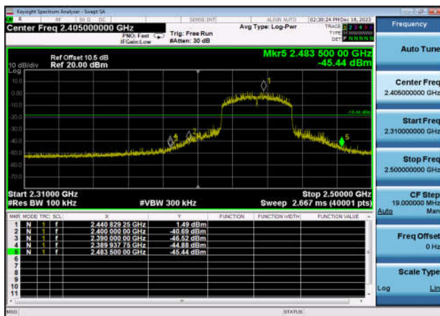
,Plot 2,Band Edge-802.11ax(HE40) ,2437MHz,Ant0
