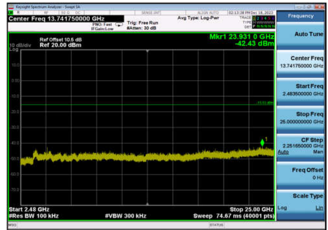
,Plot 4,2483.5MHz~25000MHz-802.11ax(H E40),2422MHz,Ant0
