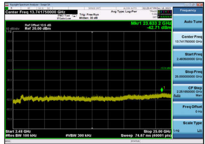
,Plot 4,2483.5MHz~25000MHz-802.11ax(H E40),2452MHz,Ant0
