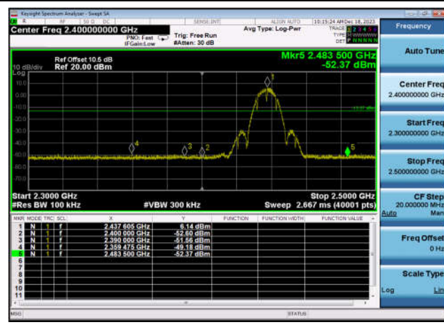
,Plot 2,Band Edge-802.11b,2437MHz ,Ant0
