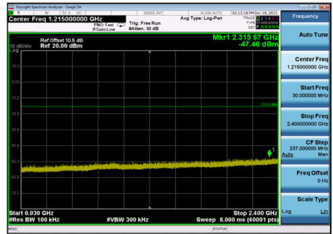
,Plot 3,30MHz~2400MHz-802.11ax(HE40) ,2422MHz,Ant0
