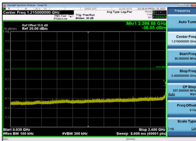
,Plot 3,30MHz~2400MHz-802.11ax(HE40) ,2437MHz,Ant0
