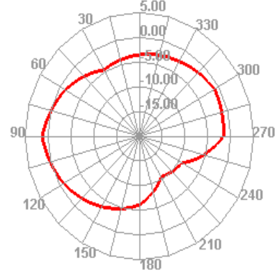
2500.000MHz E2
