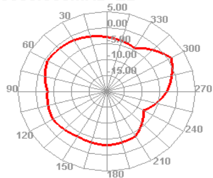
5500.000MHz E2
