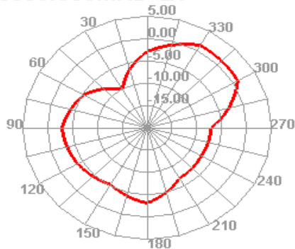
5500.000MHz E1
