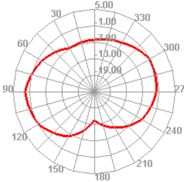
2400.000MHz H
