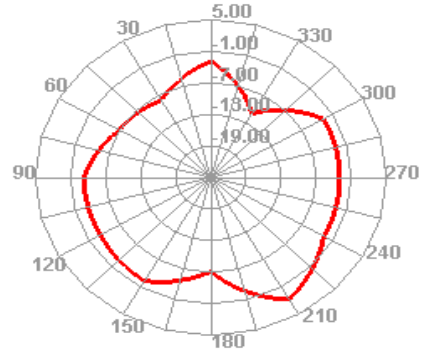
5500.000MHz H
