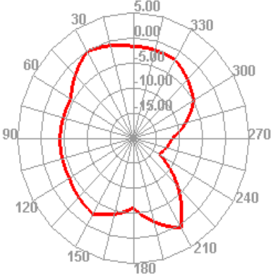
2500.000MHz E1
