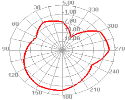
5500.000MHz E2
