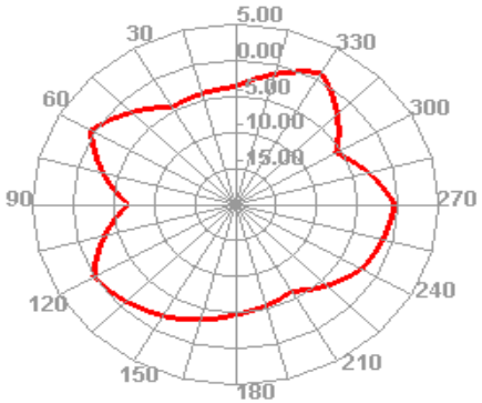
5850.000MHz E2
