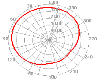
2450.000MHz H
