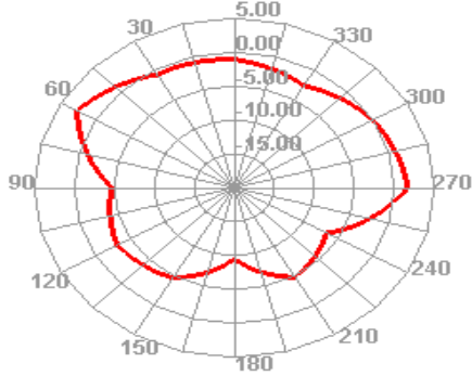
5850.000MHz H
