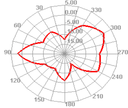
2450.000MHz H
