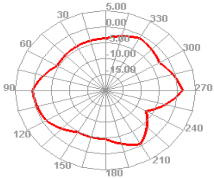
5850.000MHz E1
