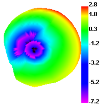
2400.000MHz E1
