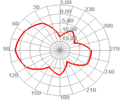
2450.000MHz
