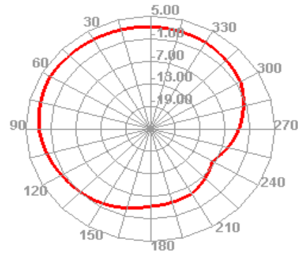
2400.000MHz E2
