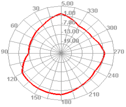
5850.000MHz H
