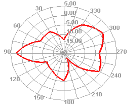
2450.000MHz E2
