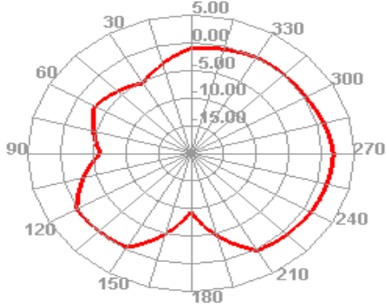
5850.000MHz
