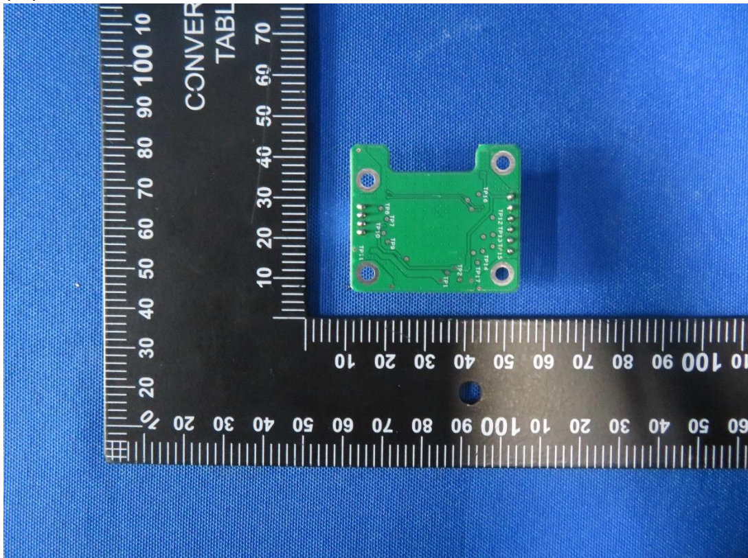
(14) EUT Photo
