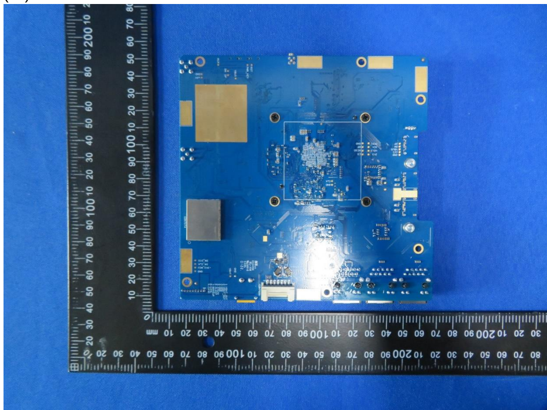
(10) EUT Photo
