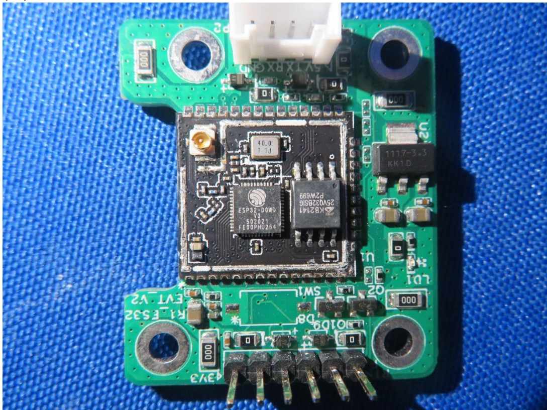
(15) EUT Photo
