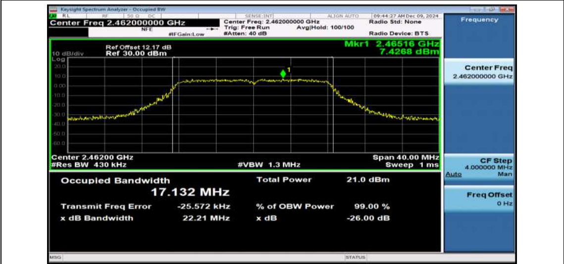
11G-Ant1-2462
