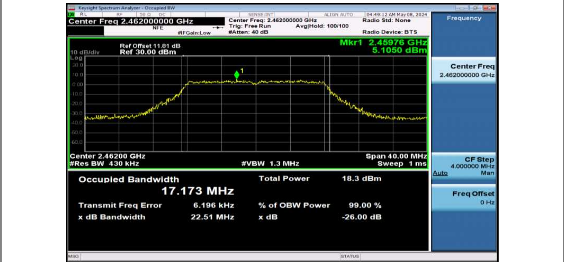
11G-Ant1-2462
