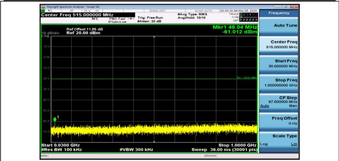
11G-Ant1-2412-30~1000-PASS
