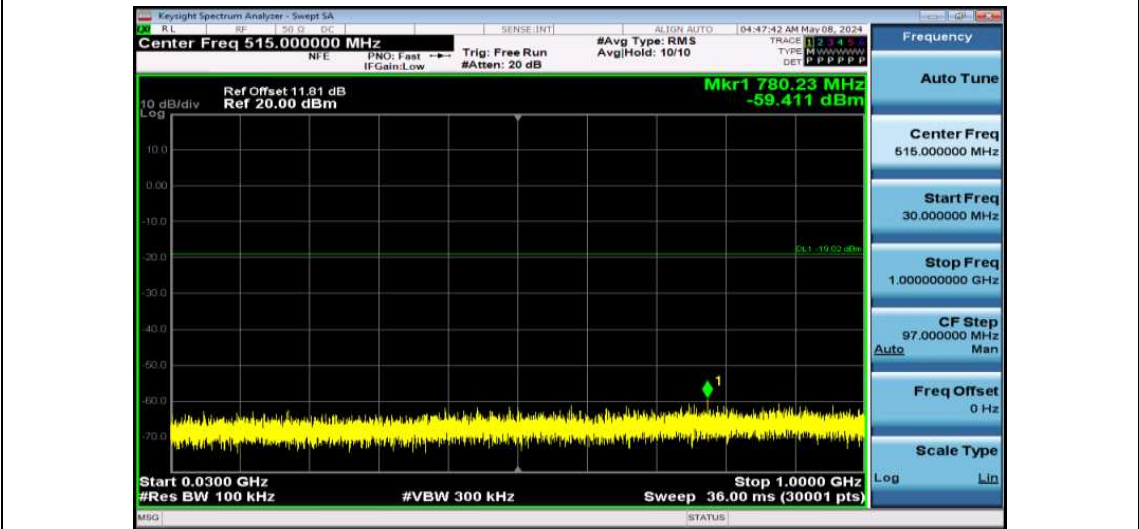
11G-Ant1-2437-30~1000-PASS
