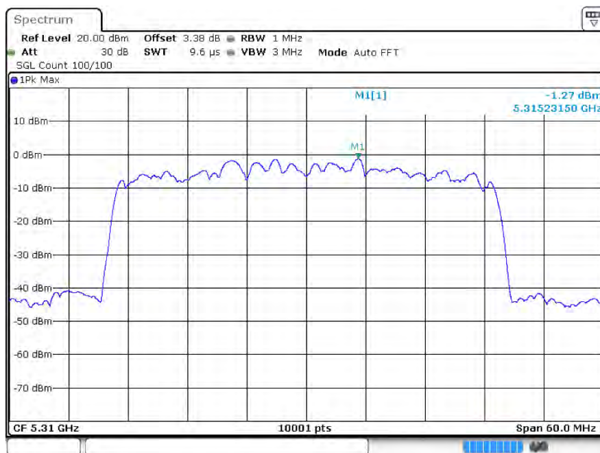
PSD ax40 5310MHz Ant2
