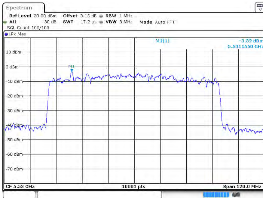
PSD ax80 5530MHz Ant1
