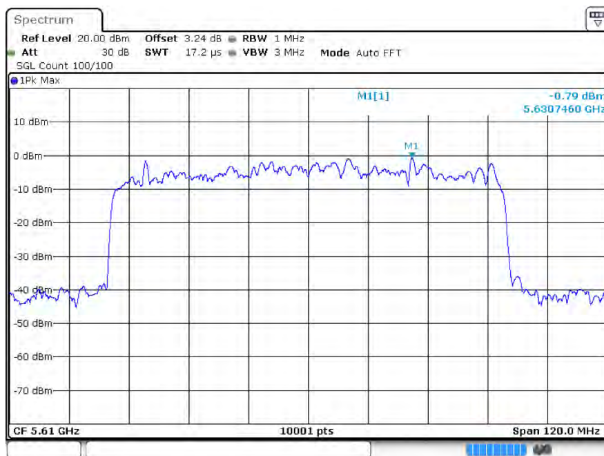
PSDax80 5610MHz Ant2
