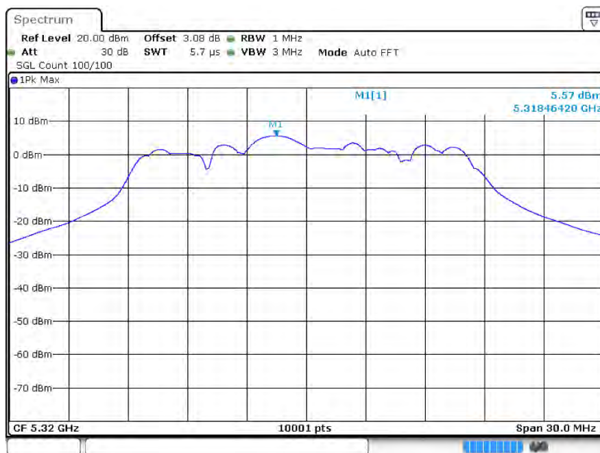
PSD ax20 5320MHz Ant1
