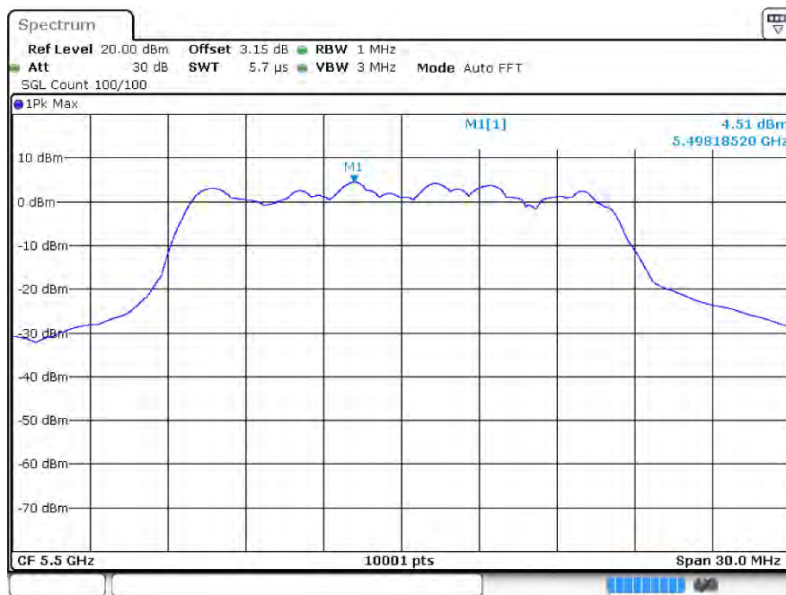
PSD ax20 5500MHz Ant2
