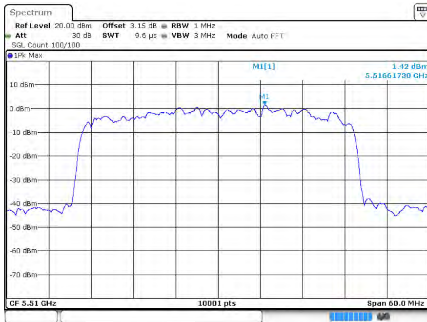
PSDax40 5510MHz Ant2
