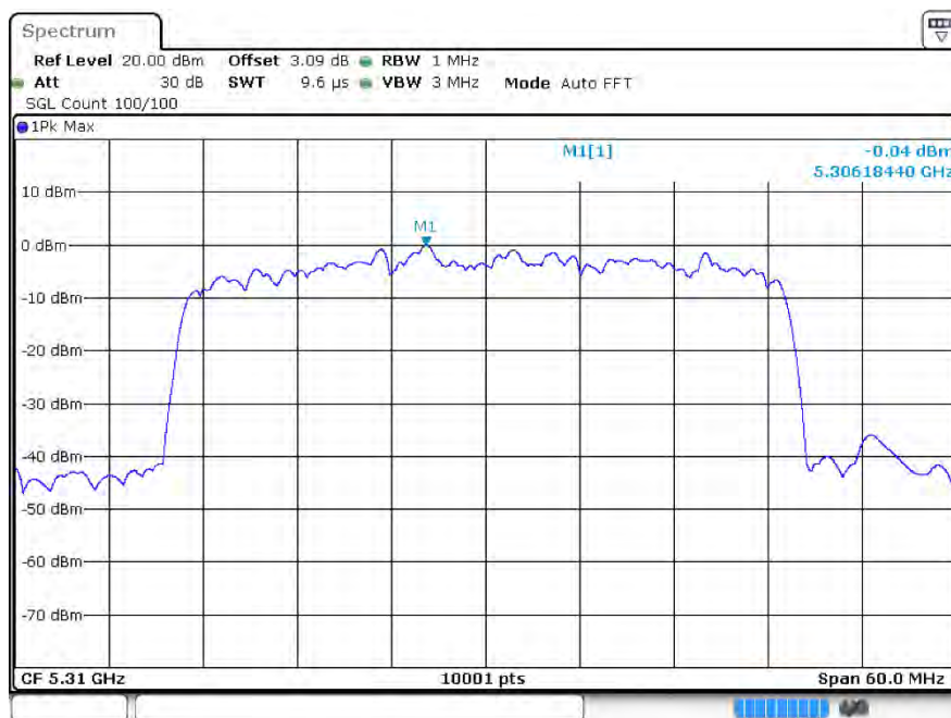
PSD ax40 5310MHz Ant1
