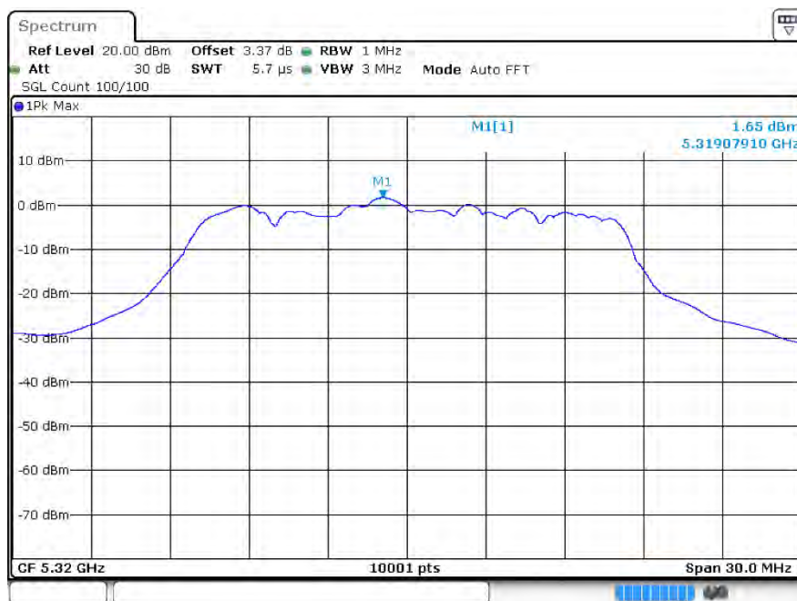
PSD ax20 5320MHz Ant2
