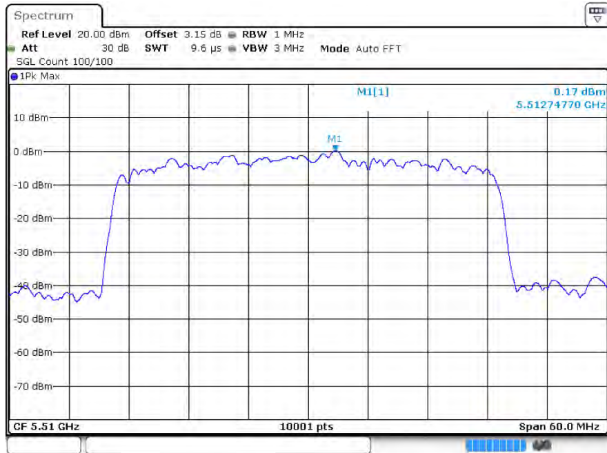
PSDax40 5510MHz Ant1
