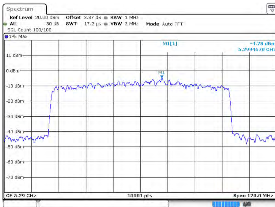
PSDax80 5290MHz Ant2
