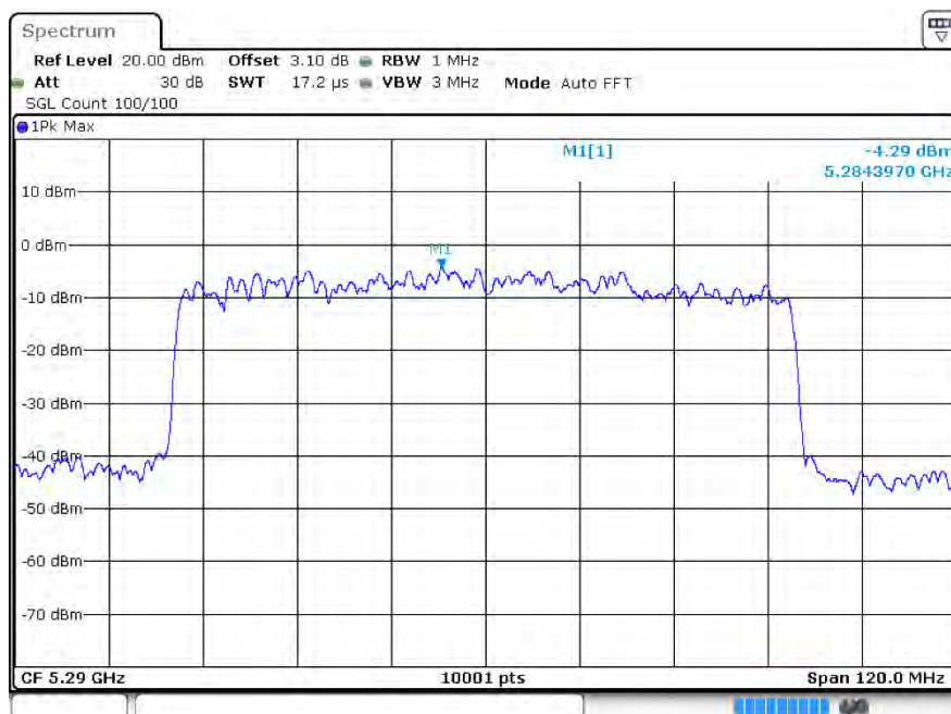
PSDax80 5290MHz Ant1
