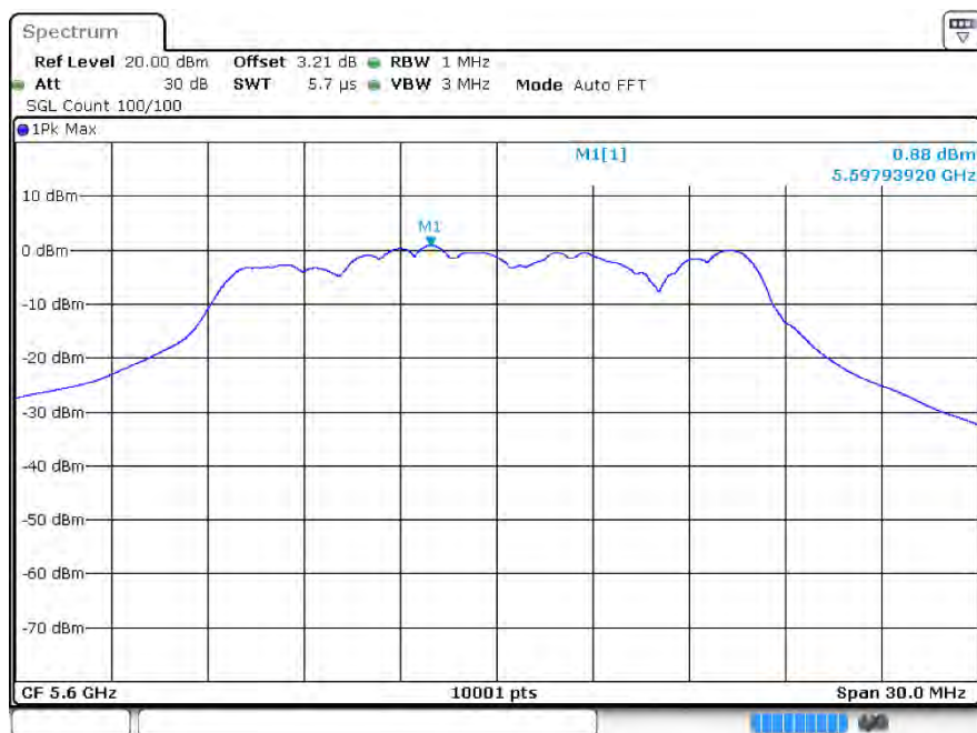
PSD ax20 5600MHz Ant1
