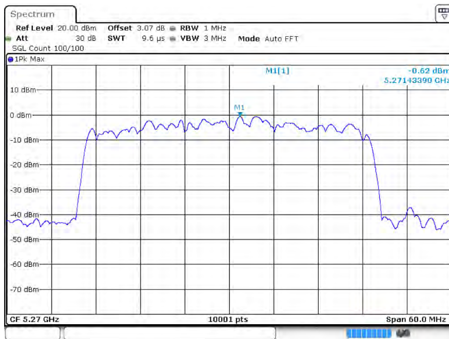
PSD ax40 5270MHz Ant1
