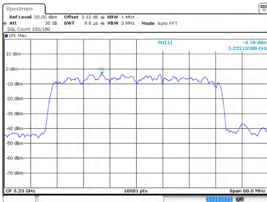
PSDax40 5230MHz Ant2
