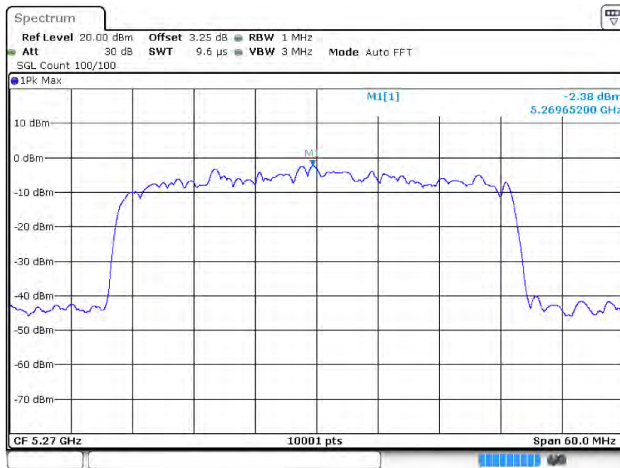
PSD ax40 5270MHz Ant2
