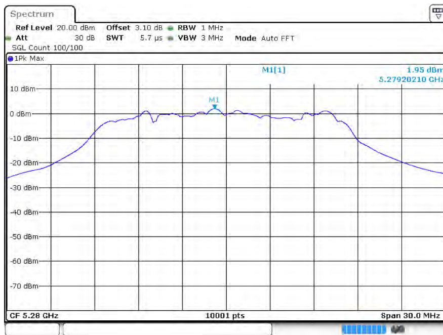
PSD ax20 5280MHz Ant1
