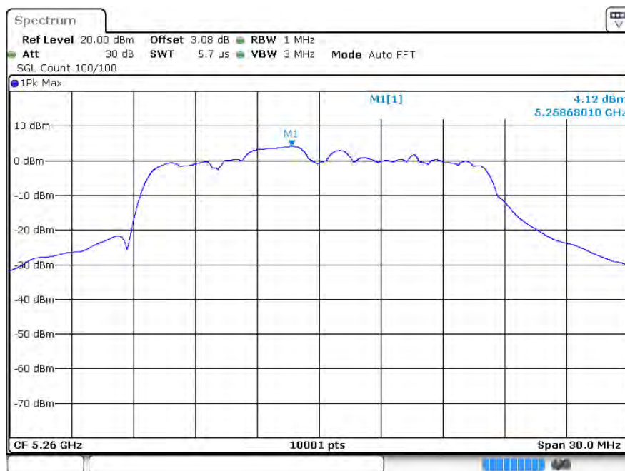
PSD ax20 5260MHz Ant1
