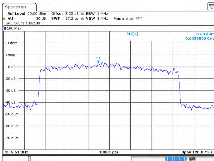
PSDax80 5610MHz Ant1
