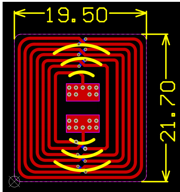
尺寸图
