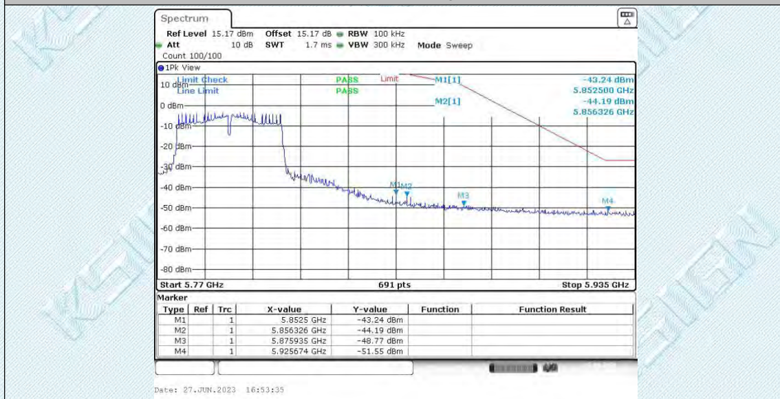
11AC80SISO_Ant1_Low_5775
