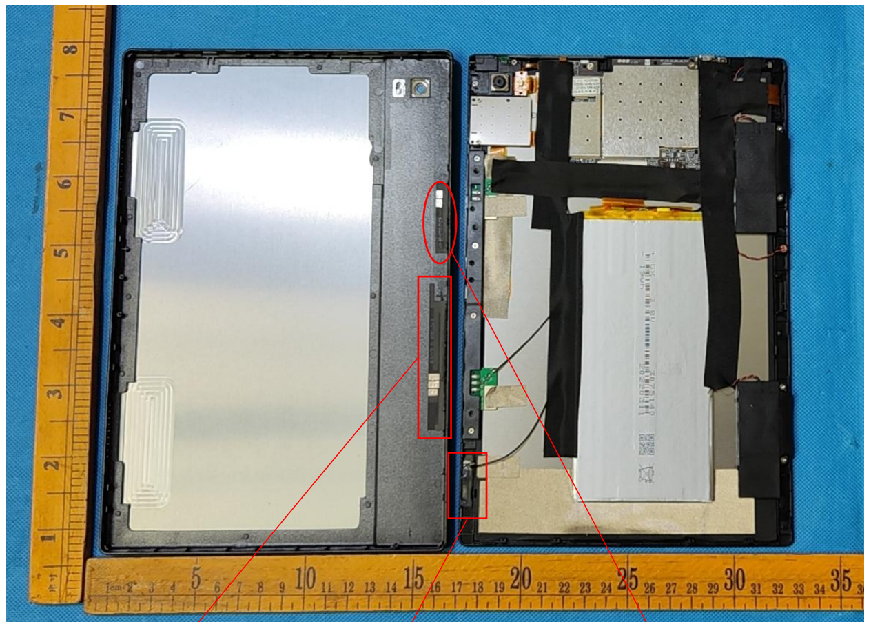
4G antenna
