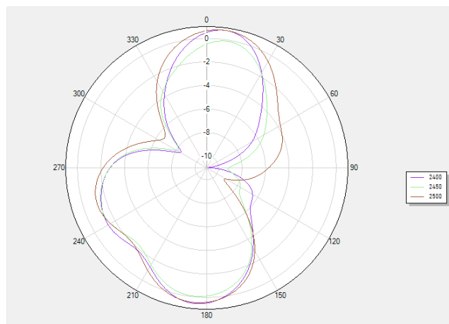
Theta 90 2D 图
