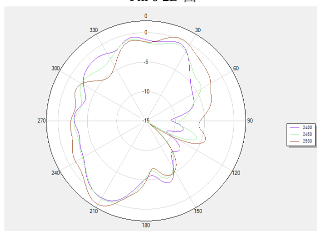
Phi 90 2D 图
