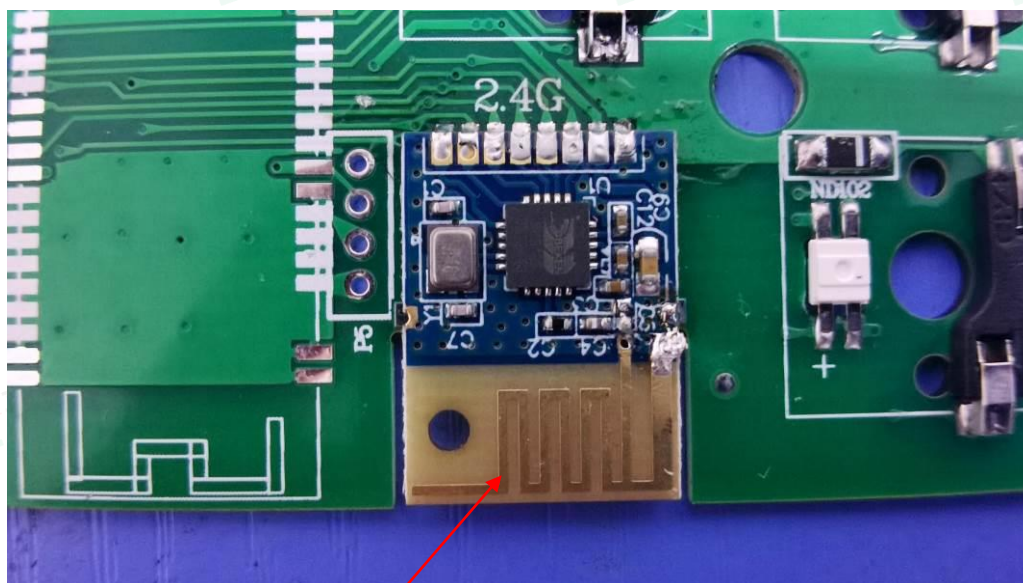
Antenna
