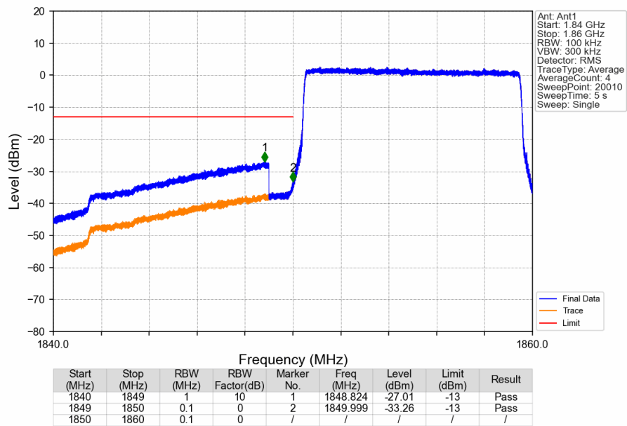
Band2_10MHz_QPSK_LCH_1855MHz_RB_50_0_NTNV
