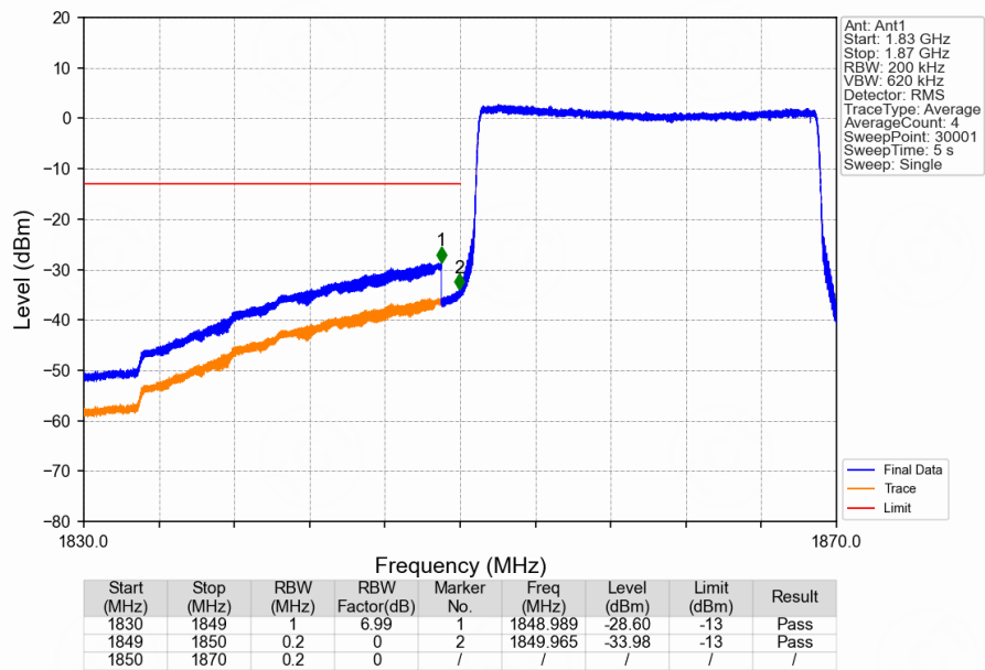
Band2_20MHz_QPSK_LCH_1860MHz_RB_100_0_NTNV
