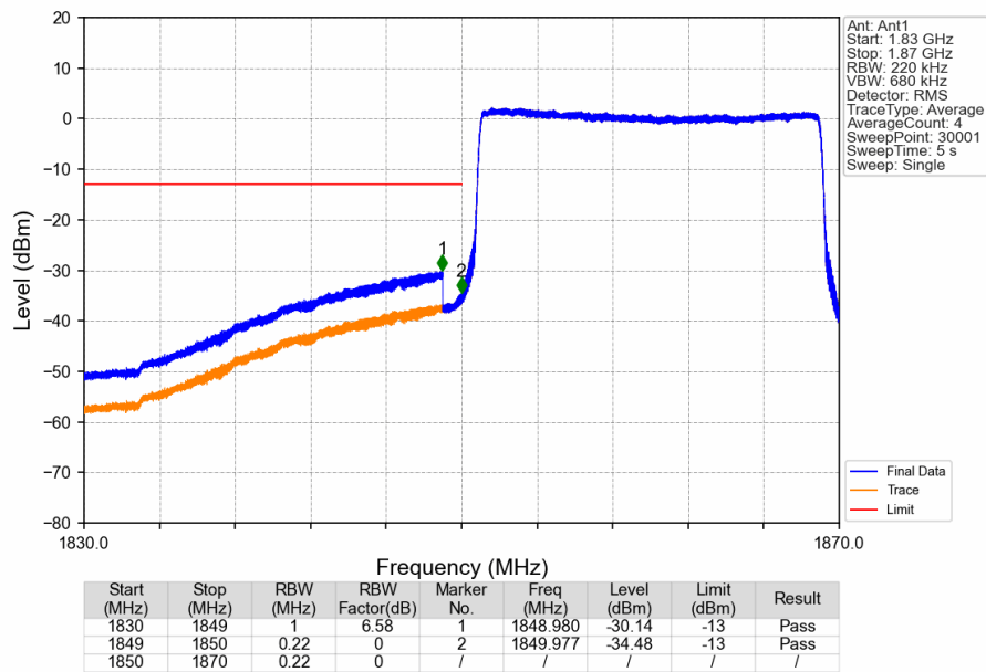
Band2_20MHz_16QAM_LCH_1860MHz_RB_100_0_NTNV
