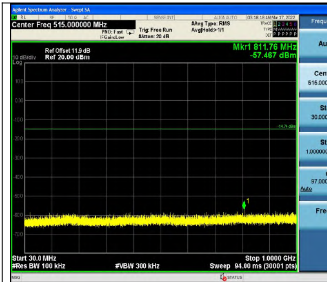
DH5_Ant1_2480_30~1000
