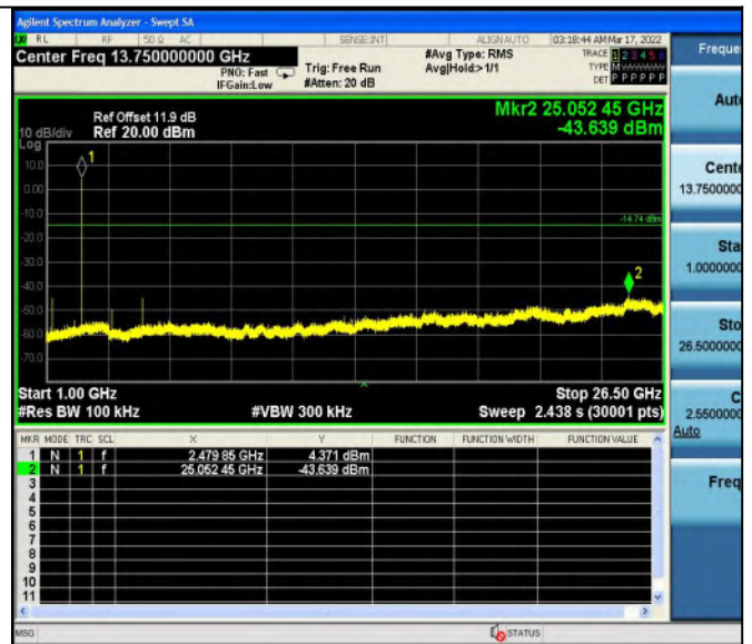
DH5_Ant1_2480_1000~26500
