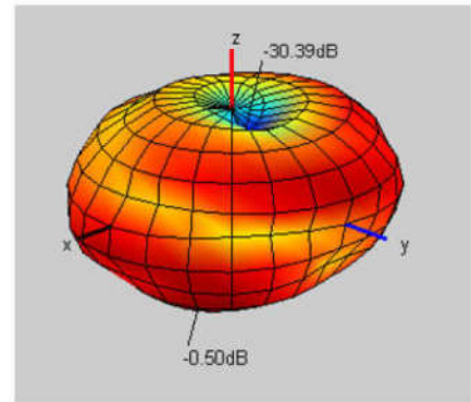
2484.000MHz
