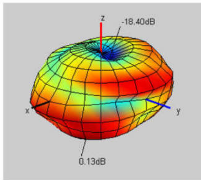
2436.000MHz
