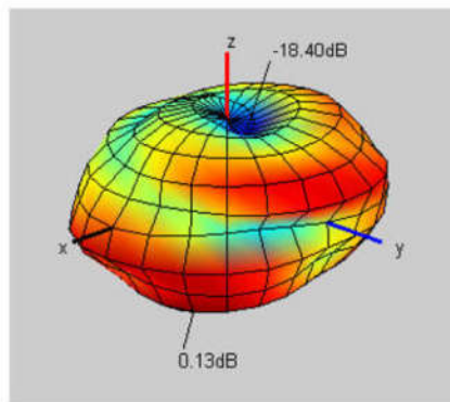
2436.000MHz
