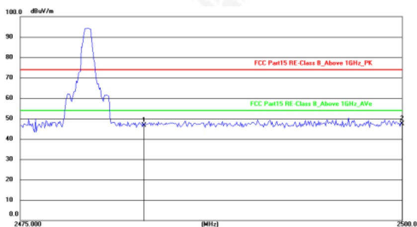
2480MHz Horizontal
