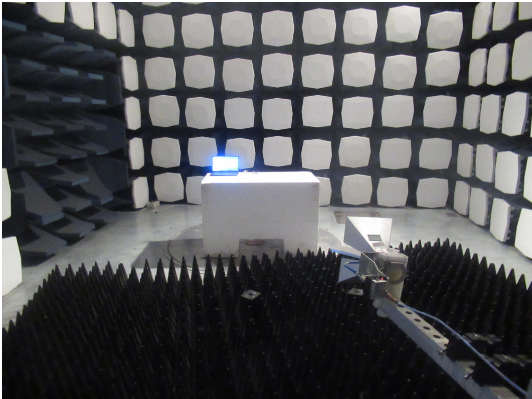
1GHz-18GHz
