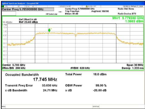
802.11ac(HT20) U-NII-3 Middle channel
