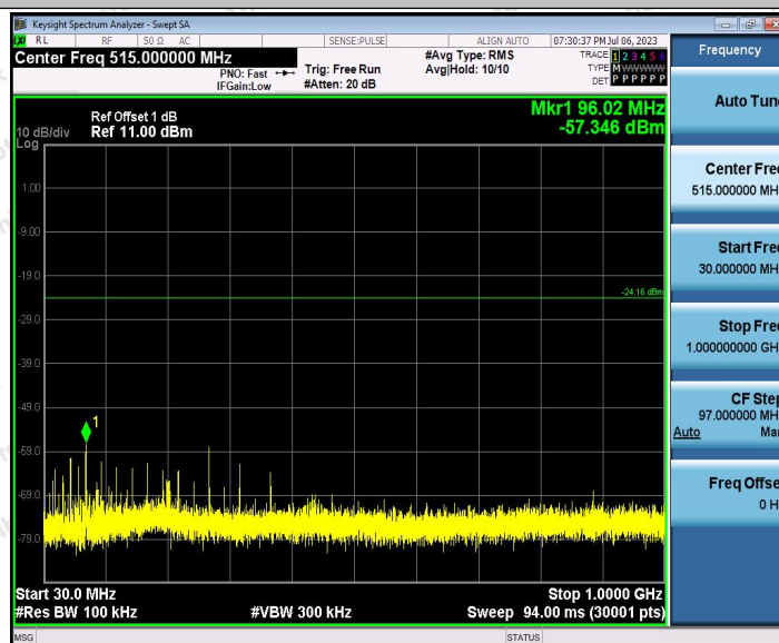
2.4G_Ant1_2439_30~1000
