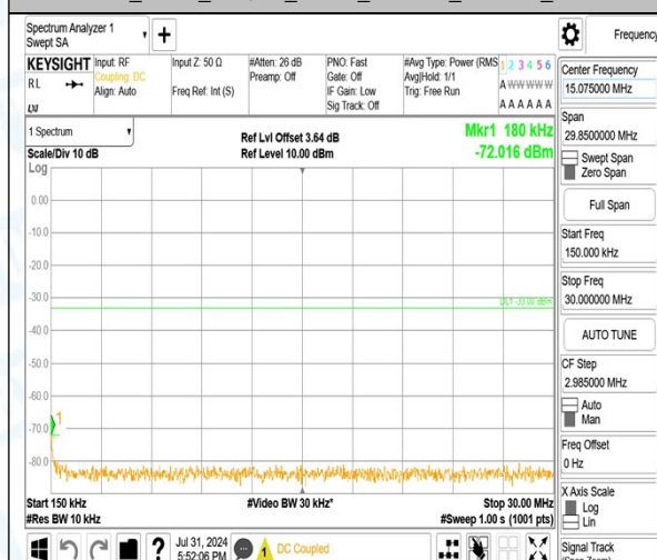
Band2 5MHz 16QAM 19175 25RB#0 0.15~30 0.15~30
