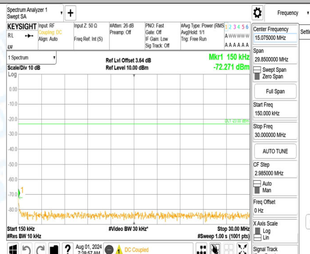
Band13 5MHz 16QAM 23230 25RB#0 1000~3000 1000~3000
