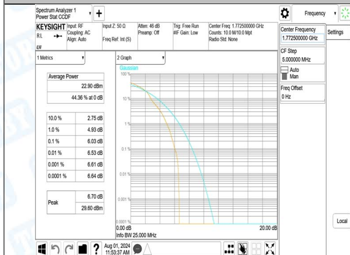
Band66-20MHz-QPSK-132072-1RB#0-PASS
