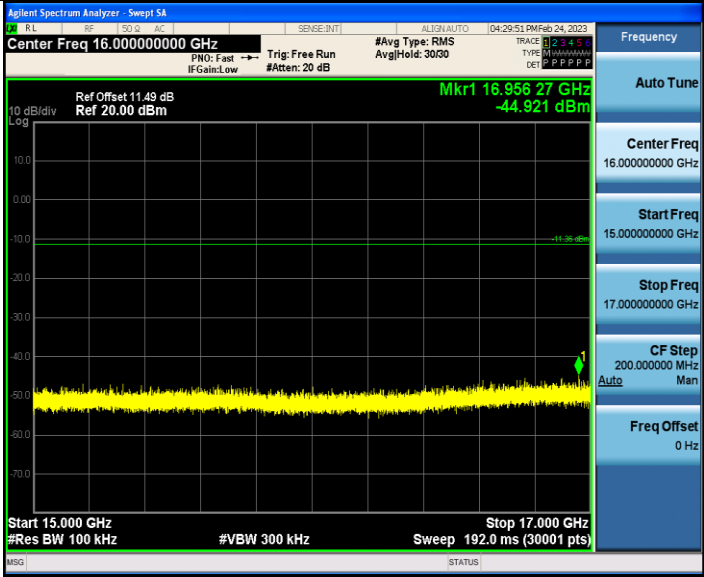
BLE_125K_Ant1_2480_15000~17000
