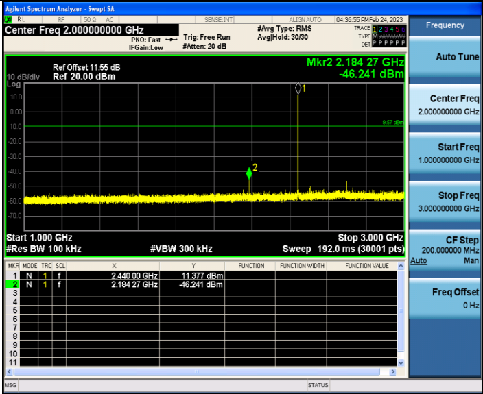
BLE_500K_Ant1_2440_1000~3000
