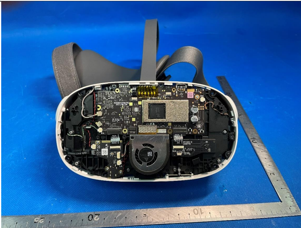
(11) EUT Photo - EUT2
