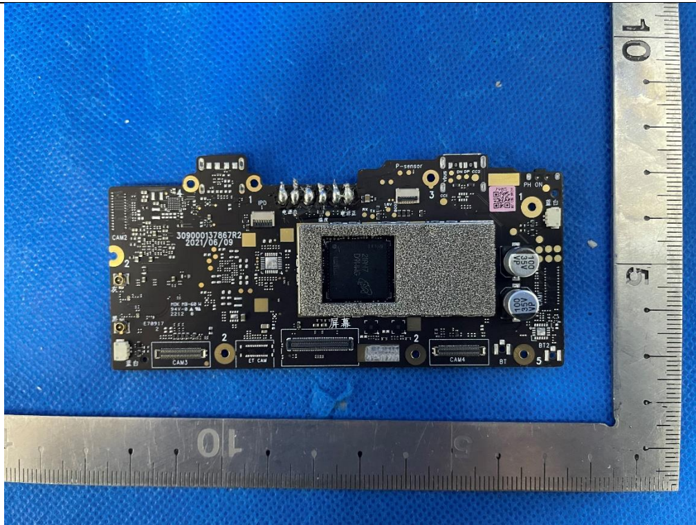
(14) EUT Photo - EUT2
