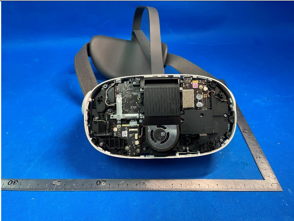
(10) EUT Photo - EUT2
