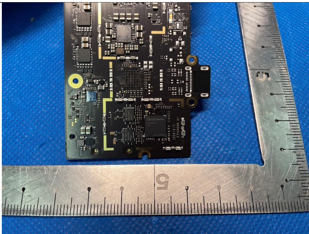
(15) EUT Photo - EUT2
