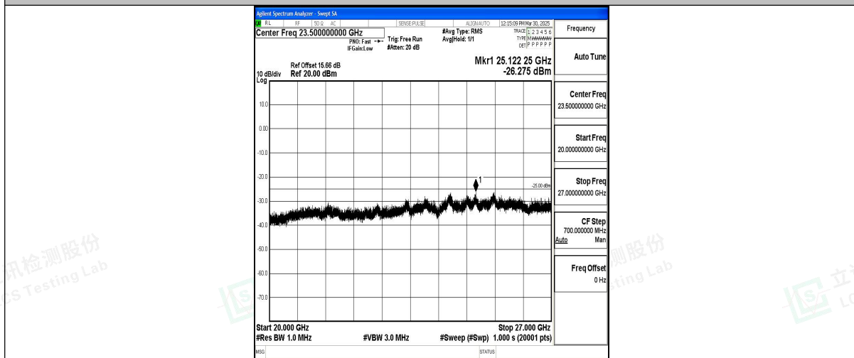
Band7_20MHz_QPSK_20850_1RB#0_20000~27000_20000~27000
