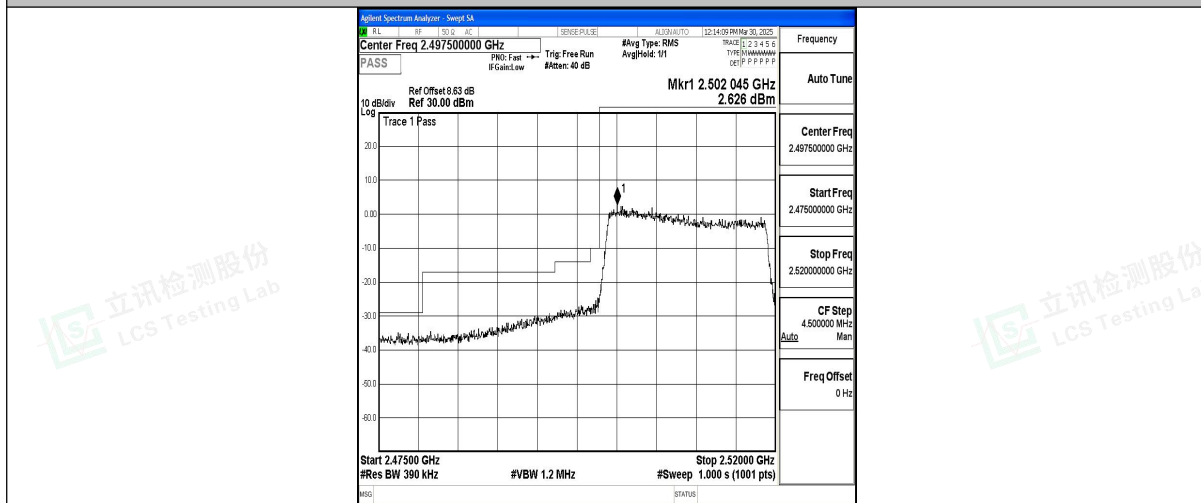
Band7_20MHz_QPSK_20850_100RB#0
