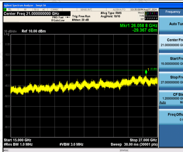
Band7-5MHz-QPSK-21425-1RB#0-Range3:15000~27000MHz
