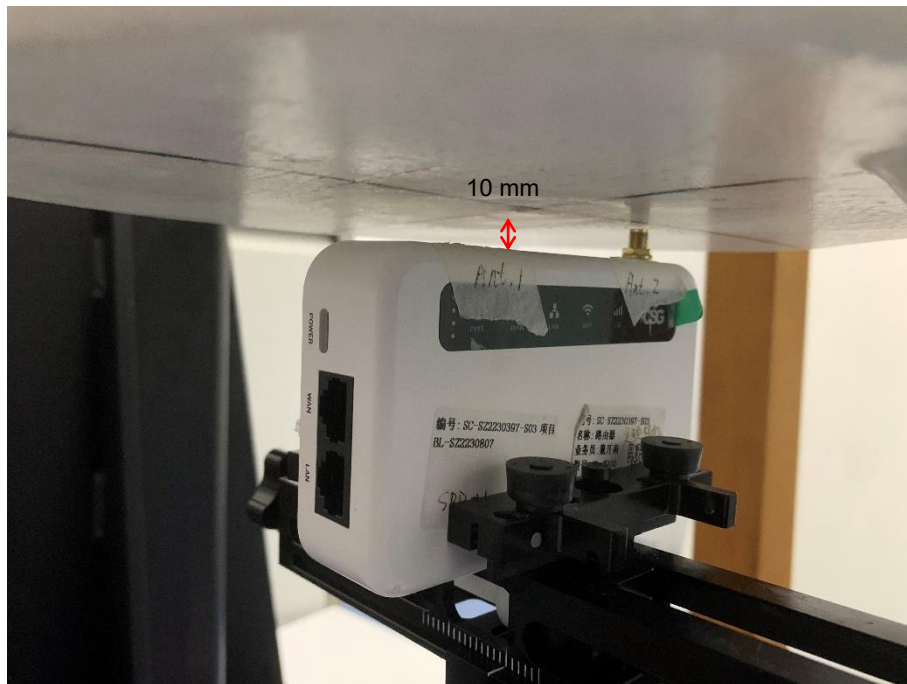
Top Edge (10mm) of WLAN Antenna
