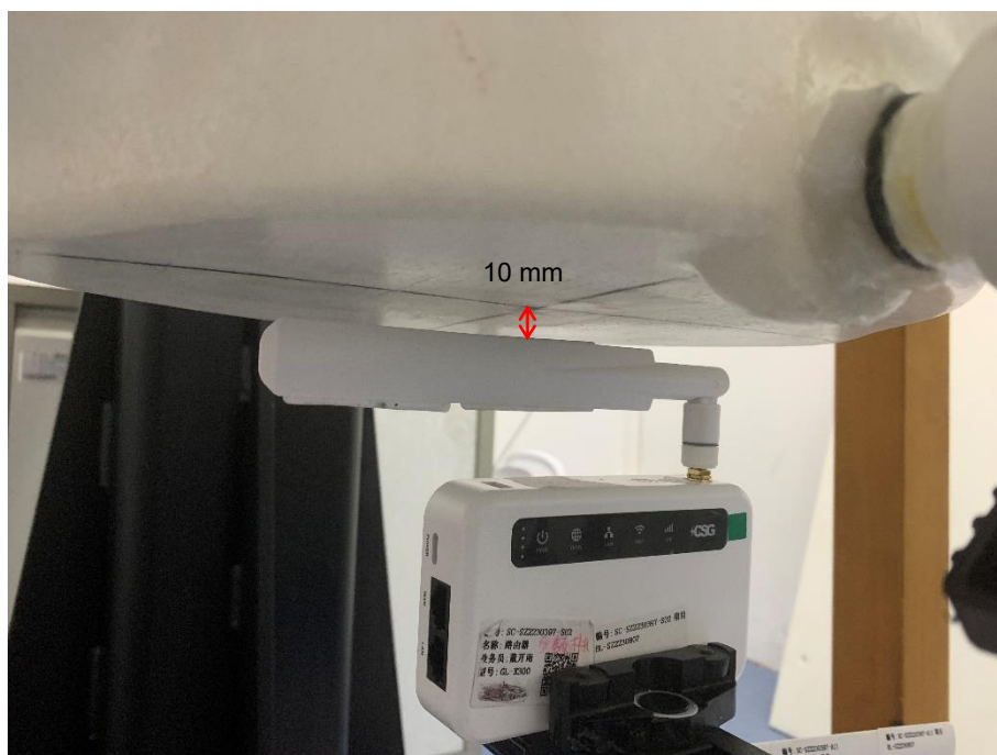
Top Edge (10mm) of WWAN Antenna
