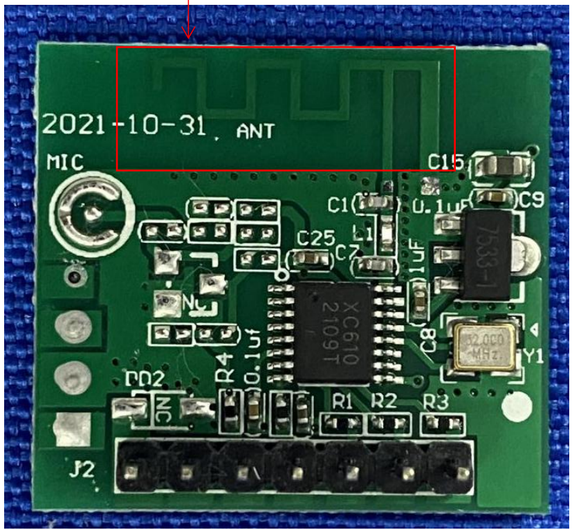
Antenna
