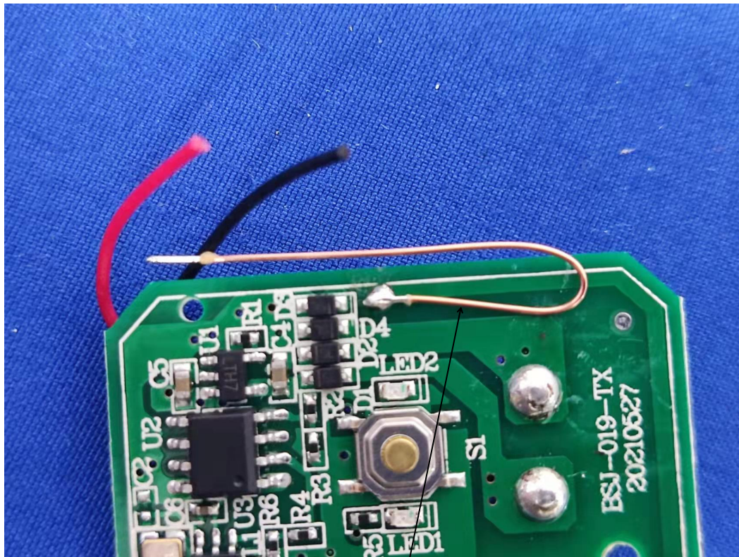
Internet Antenna
