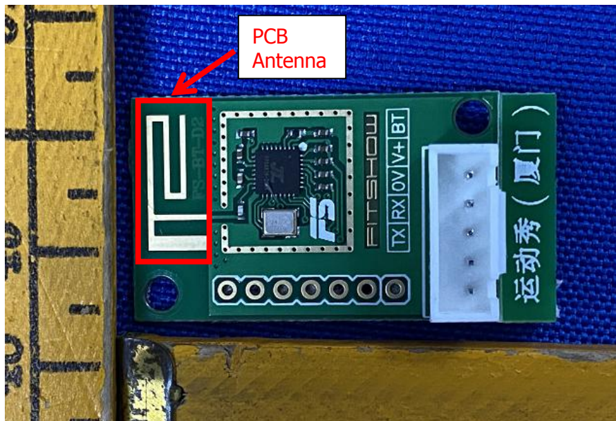
BLE Module
