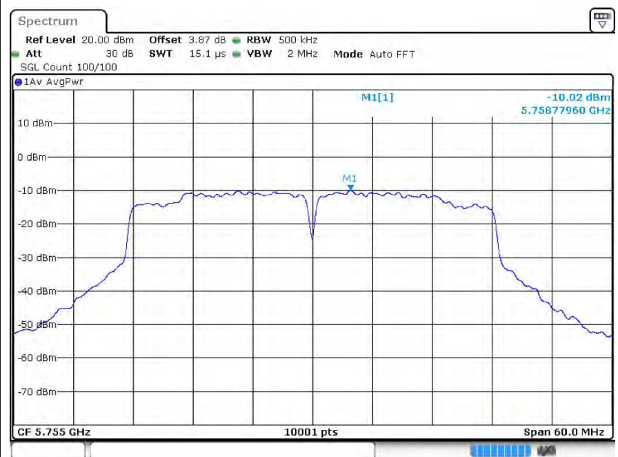
PSD ac40 5755MHz Ant1
