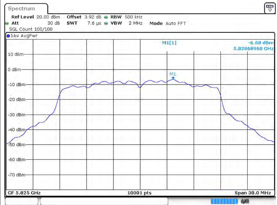
PSD ac20 5825MHz Ant1
