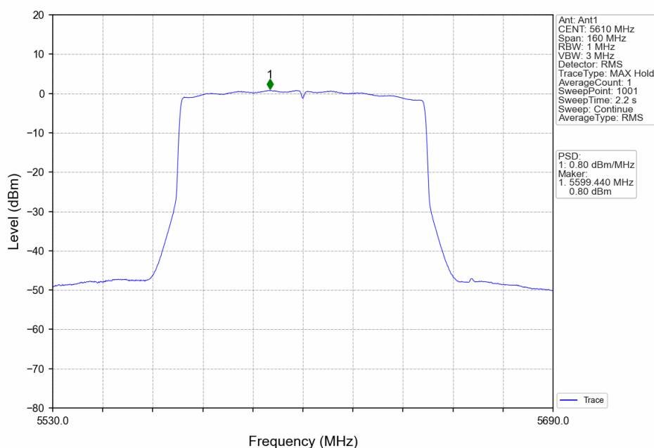
802.11ax(HEW80)_HCH_5610MHz_RU996_Left_Ant1_NTNV
