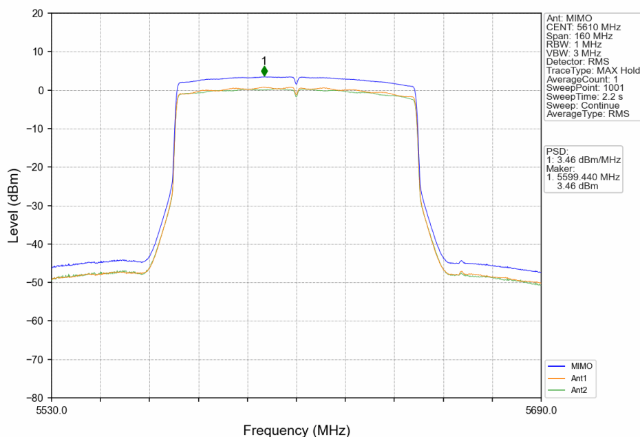
802.11ax(HEW80)_HCH_5610MHz_RU996_Left_MIMO_NTNV
