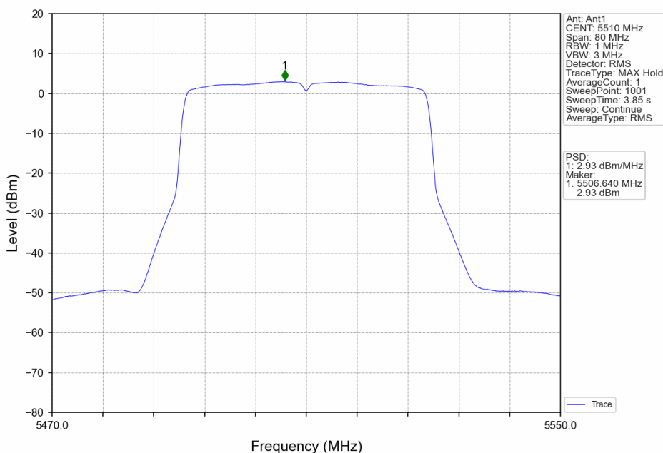
802.11ax(HEW40)_LCH_5510MHz_RU484_Left_Ant1_NTNV
