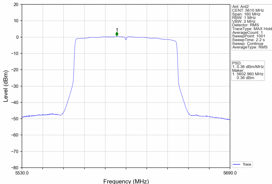
802.11ax(HEW80)_HCH_5610MHz_RU996_Left_MIMO_NTNV
