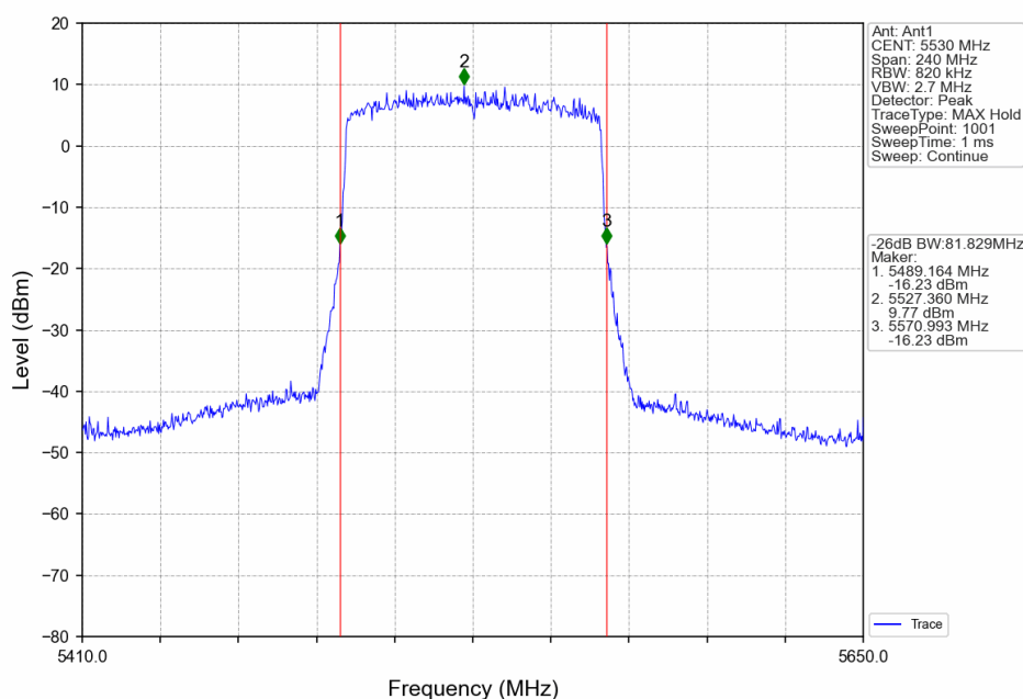
802.11ax(HEW80)_LCH_5530MHz_RU996_Left_Ant1_NTNV
