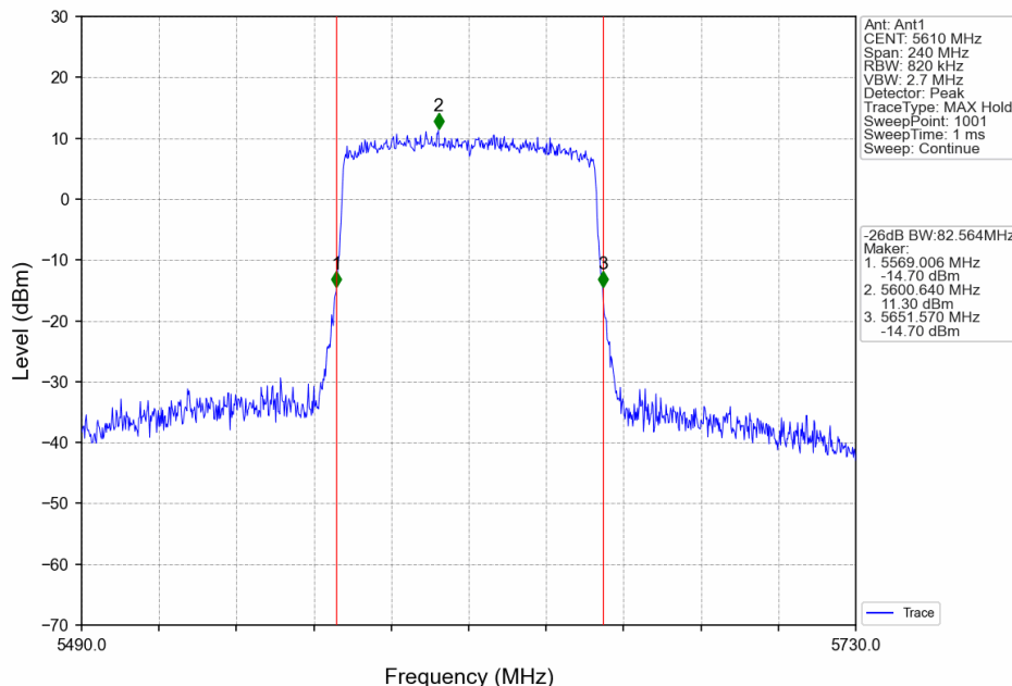
802.11ax(HEW80)_HCH_5610MHz_RU996_Left_Ant1_NTNV
