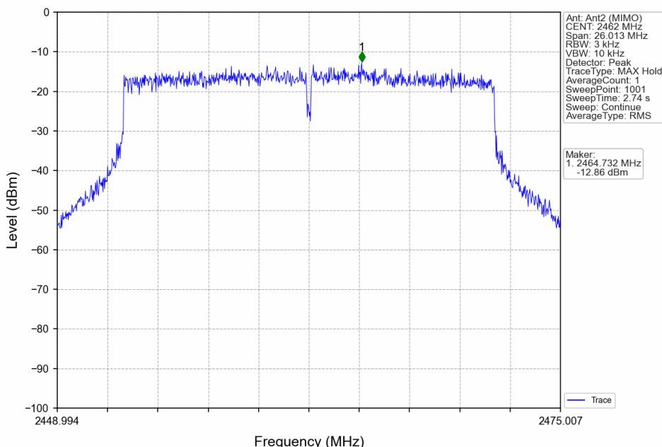
802.11ax(HEW20)_HCH_2462MHz_RU242_Left_Ant2 (MIMO)_NTNV
