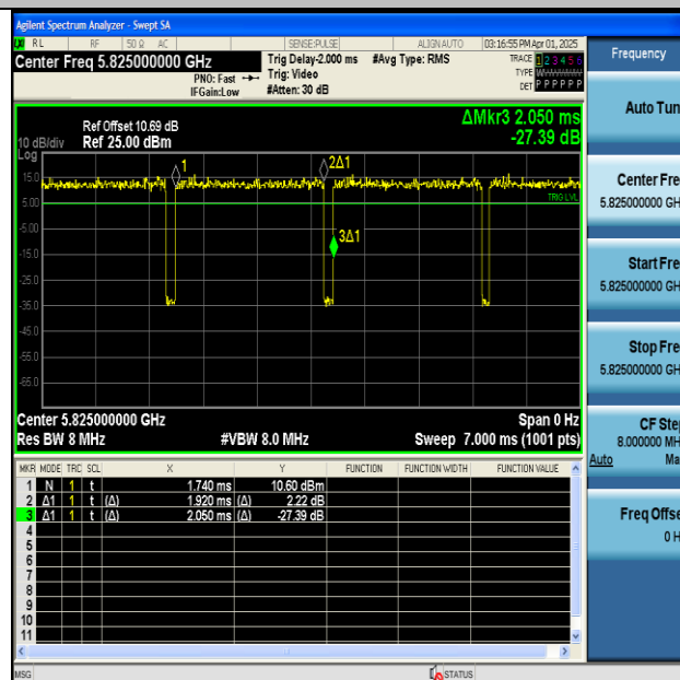
NTNV-11N20MIMO-Ant1-5825
