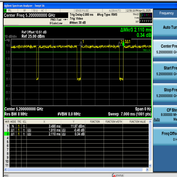
NTNV-11N20MIMO-Ant2-5200
