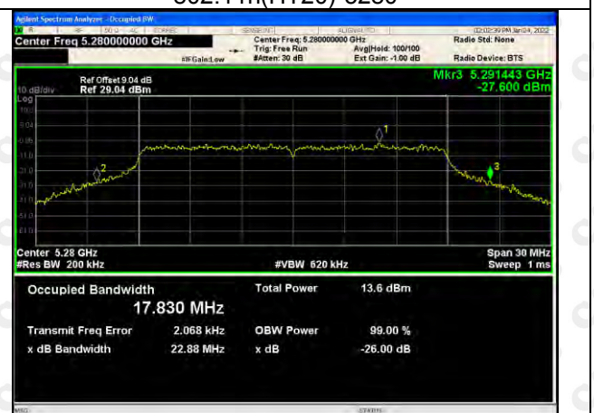
802.11n(HT20)-5280
